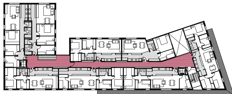
PLANTA PRIMERA
