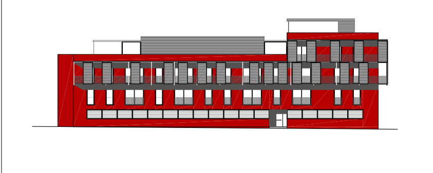
ALÇAT A-A'
