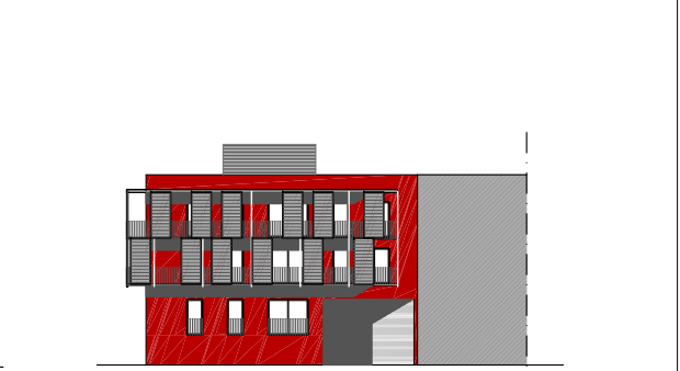
ALÇAT C-C'
