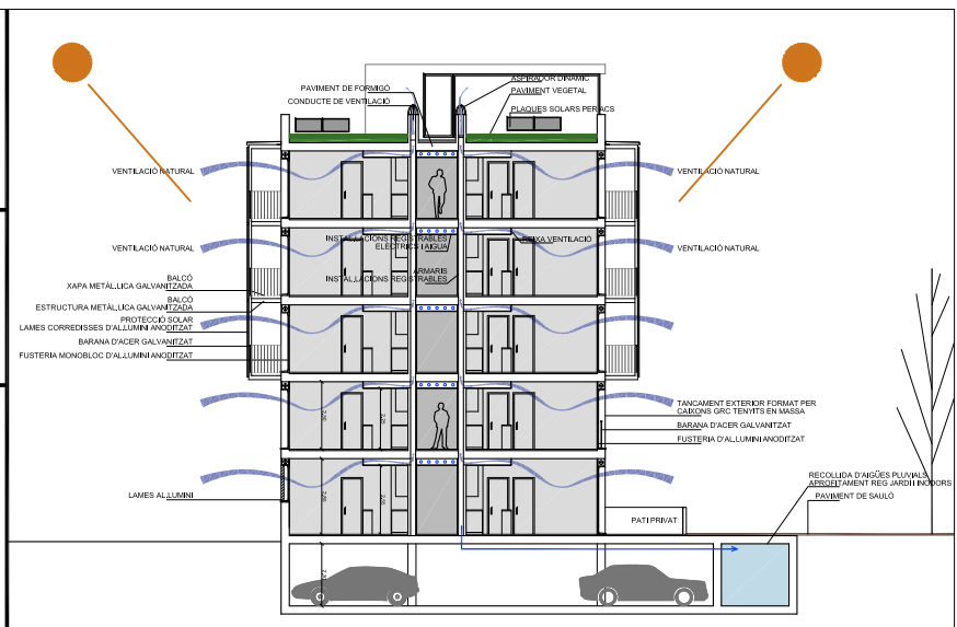
FUNCIONAMENT EDIFICI
